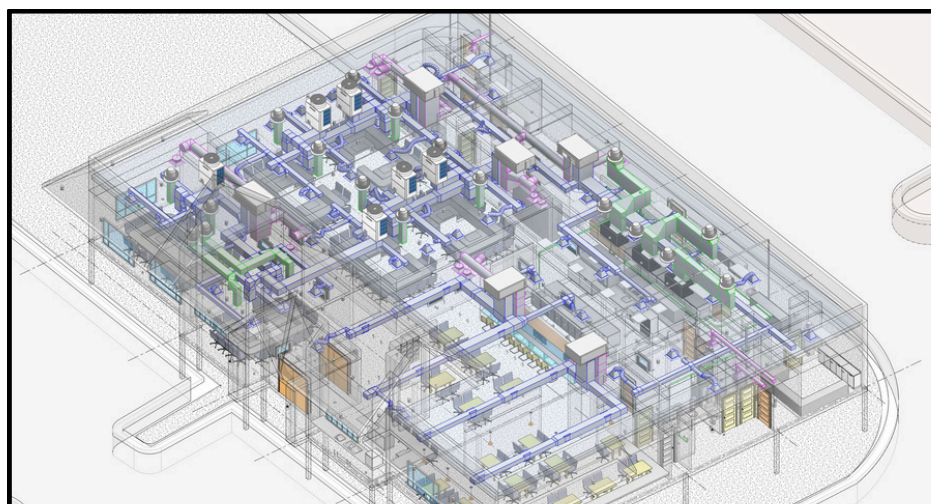
MEP BIM
